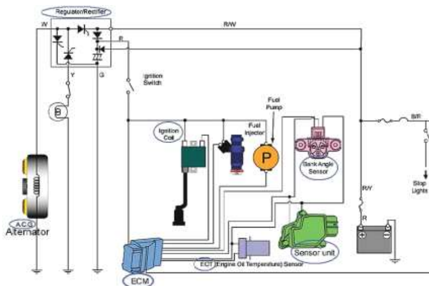
Gambar 2. skema kontrol elektronik cbr 150.
