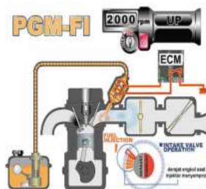
Gambar 4. ilustrasi penyemprotan pada 2000 rpm.
