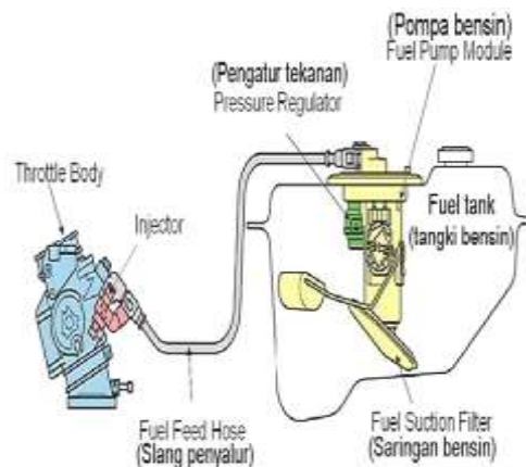
Gambar 1. skema aliran bahan bakar.
