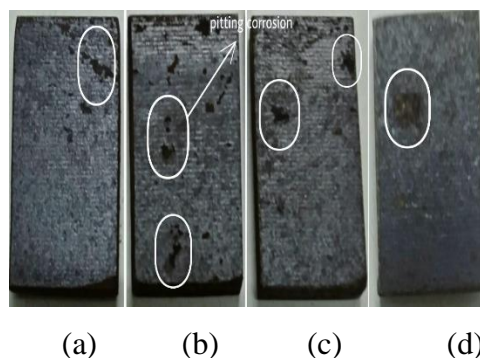
Gambar 3. Spesimen (a), (b), (c) dan (d) sesudah diuji larutan NaOH
