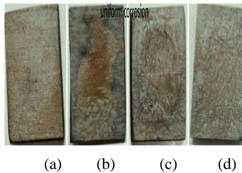
Gambar 2 Spesimen (a), (b), (c) dan (d) sesudah diuji larutan HCl
