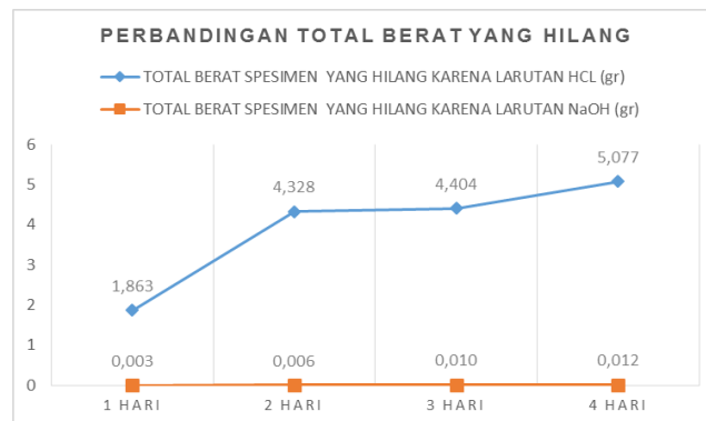
Gambar 8. Perbandingan total kehilangan berat spesimen yang sudah diuji dilarutan HCl dan NaOH
