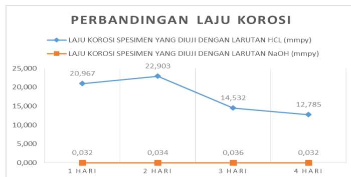
Gambar 9. Perbandingan laju korosi pada spesimen yang sudah diuji dilarutan HCl dan NaOH
