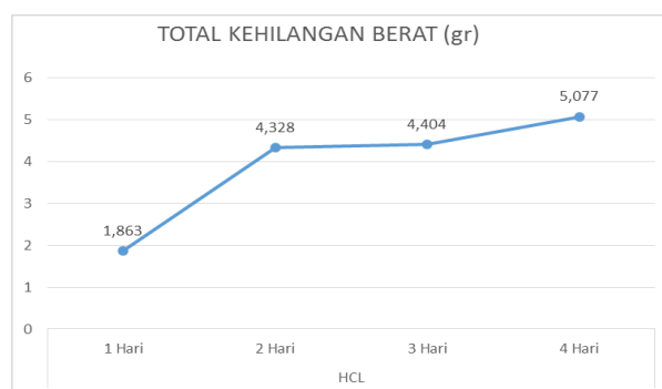
Gambar 4. Total kehilangan berat spesimen yang sudah diuji larutan HCl
