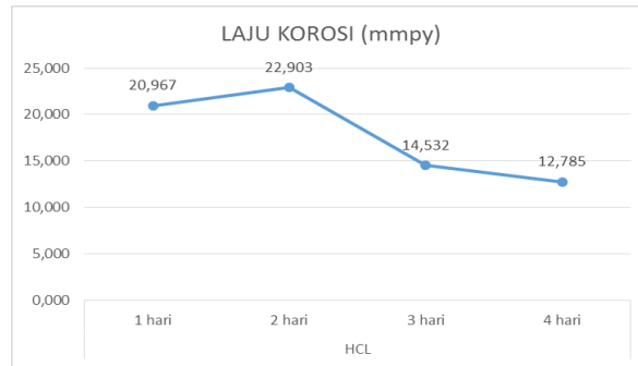
Gambar 5. Laju korosi pada spesimen yang sudah diuji larutan HCl
