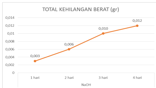
Gambar 6. Total kehilangan berat spesimen yang sudah diuji larutan NaOH
