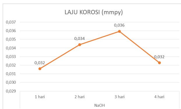
Gambar 7. Laju korosi pada spesimen yang sudah diuji larutan NaOH
